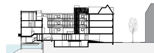
Doorsnede BB'
